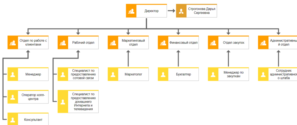
Рисунок 7 – Организационная модель
