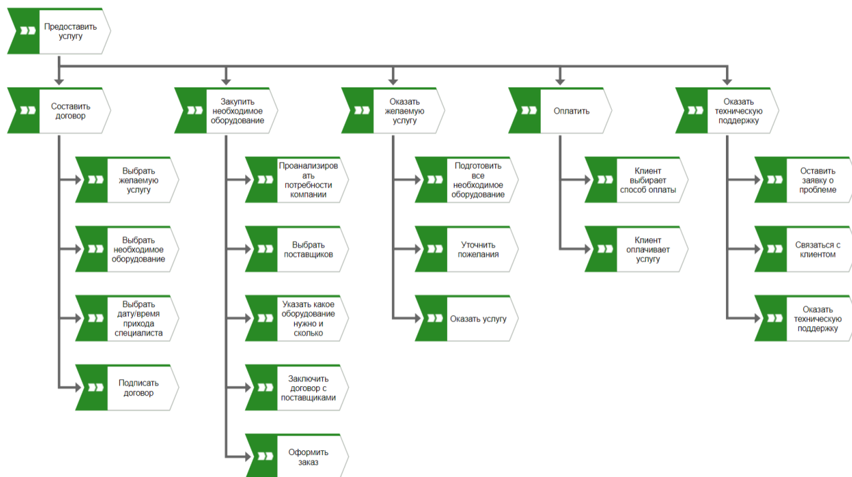
Рисунок 9 – Модель функций
