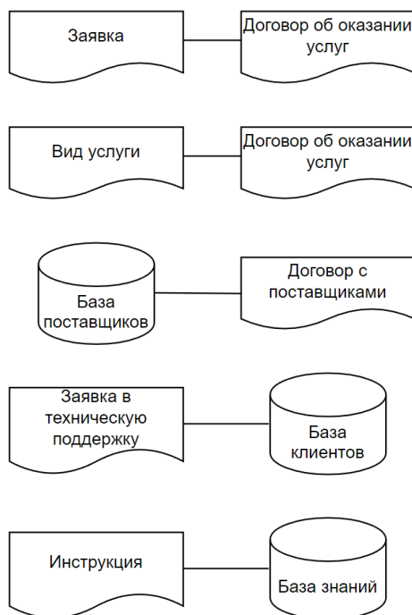
Рисунок 10 – Модель «Входов-Выходов»
