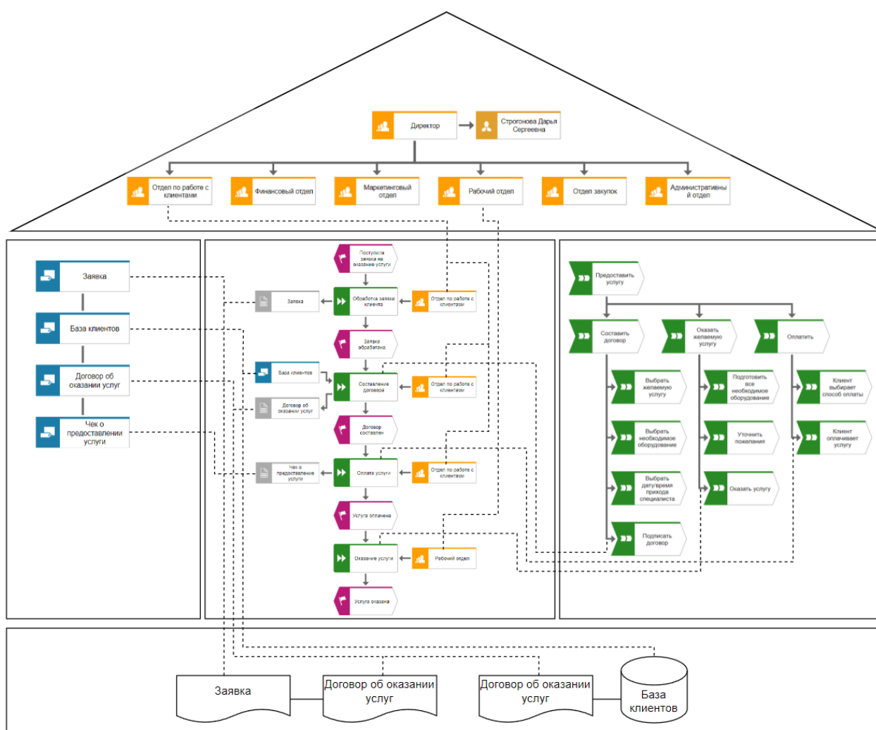
Рисунок 16 – Дом ARIS
